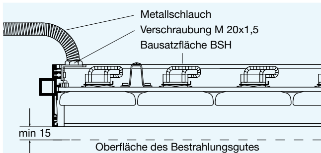
Bild 5: Anordnung der Anschlusseinheit zur Herstellung des Netzanschlusses. Abmessungen in mm
